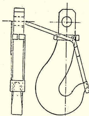
Fig. 5 - Gancio per secchioni per acciaio fuso, F. Krupp, Rheinhausen.
