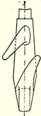
Fig. 1 - Gancio della Maschinenfabrik Duisburg.
