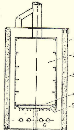
1 - camera di riscaldamento; 2 - camera di essiccazione; 3 - isolante; 4 - lamiera di distribuzione dell'aria; 5 - lamiera di fondo; 6 - fori per i bruciatori.
