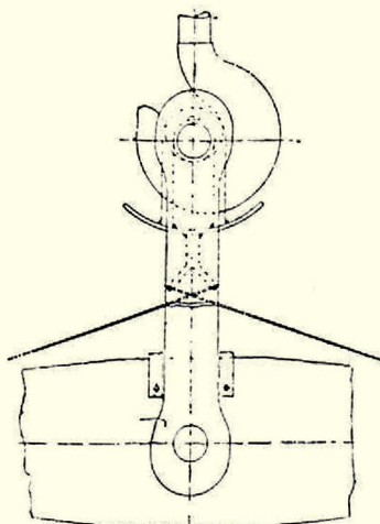
Fig. 6 - Gancio di sicurezza usato in alcune acciaierie.
