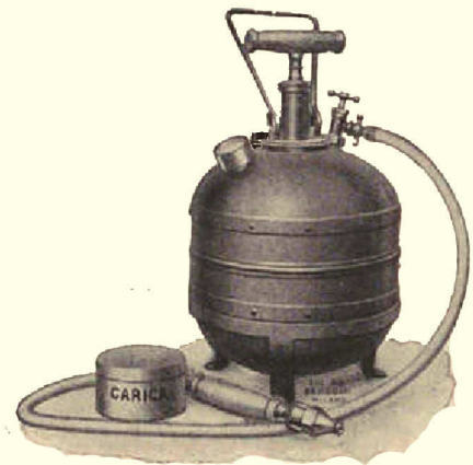
Estintore speciale per camini
